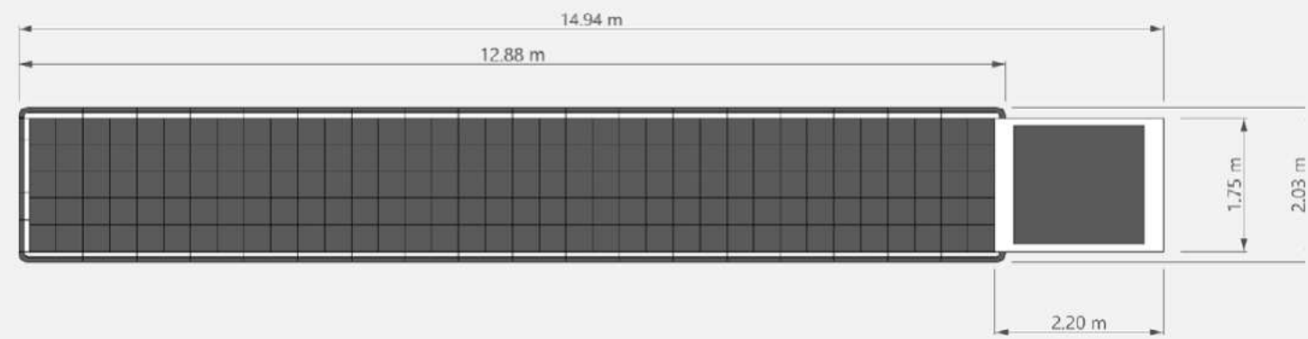
Croquis de la plateforme de bus Vectorial® avec configuration en îlot et rampe d'accès latérale.
