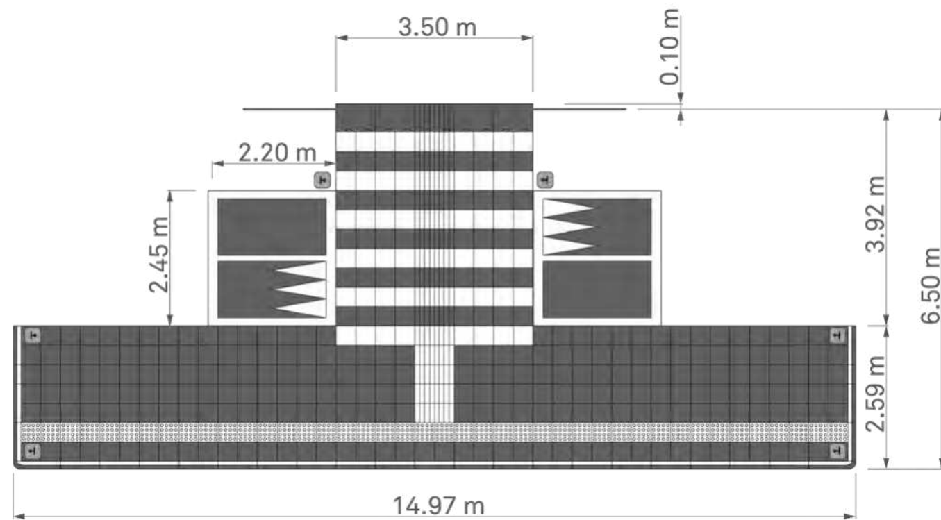
Croquis de la plateforme de bus Vectorial® avec passerelle d'accès et piste cyclable intégrée, installée rue sous les vignes.
