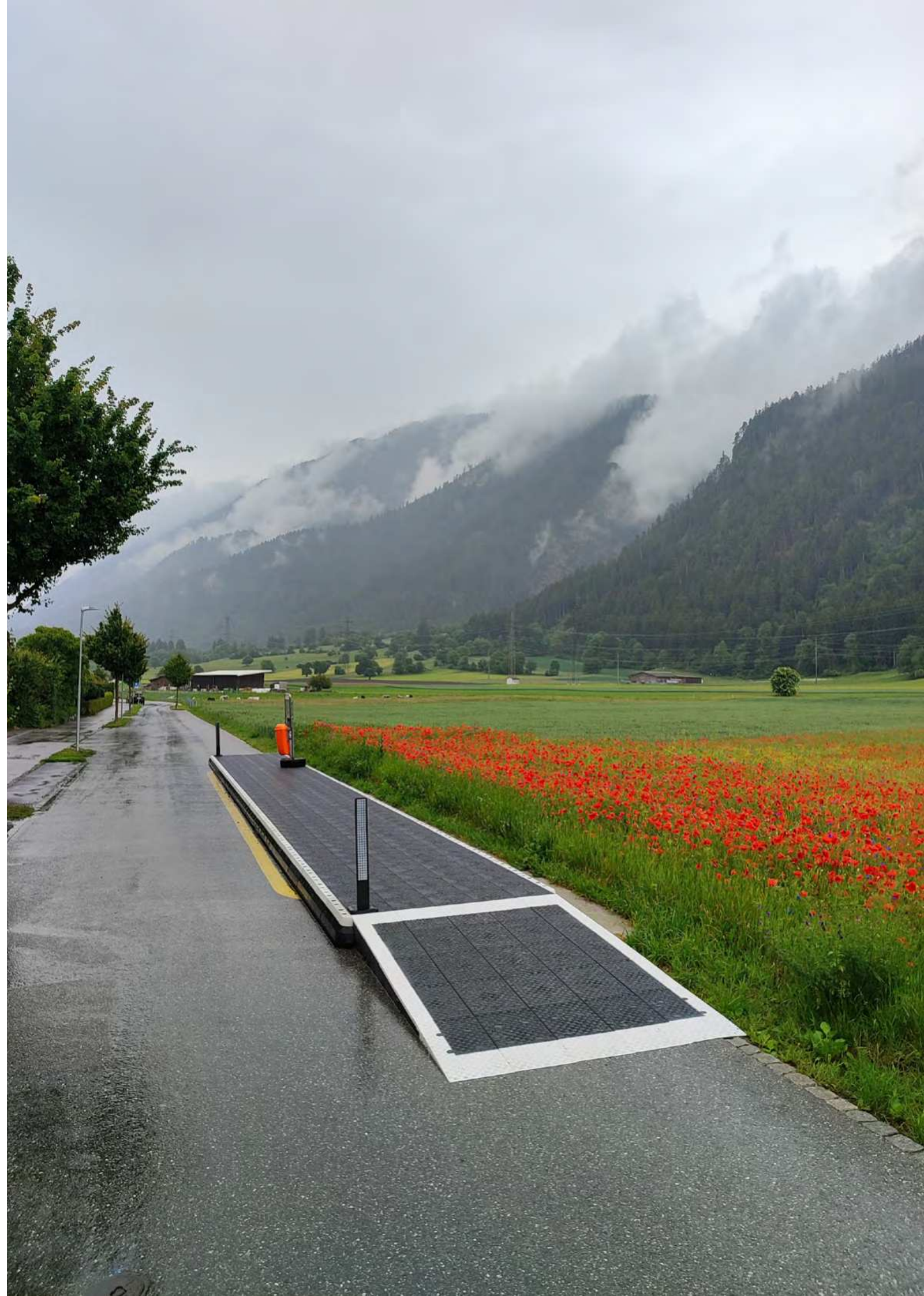
Plateforme de bus Vectorial® en configuration îlot avec deux rampes d'accès latérales et délinéateurs verticaux Pointer® Flex.
