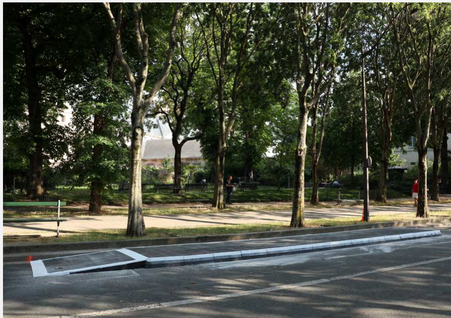
Proposition de rendu du système Vectorial® avec palier de repos pour les Jeux olympiques et paralympiques 2024.
