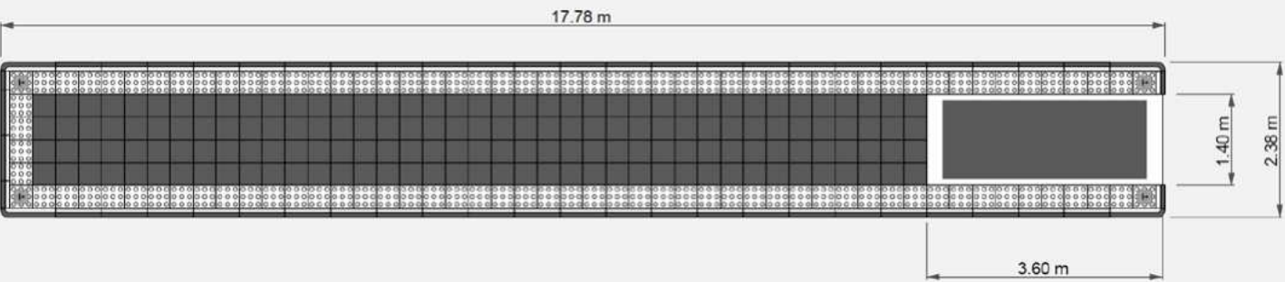
Croquis de la plateforme de bus Vectorial® avec configuration en îlot et rampe d'accès protégée.
