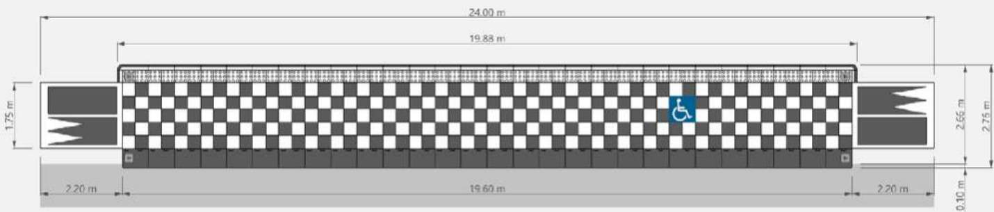
Croquis de la plateforme de bus Vectorial® avec piste cyclable intégrée, au niveau du Bd des Minimes.
